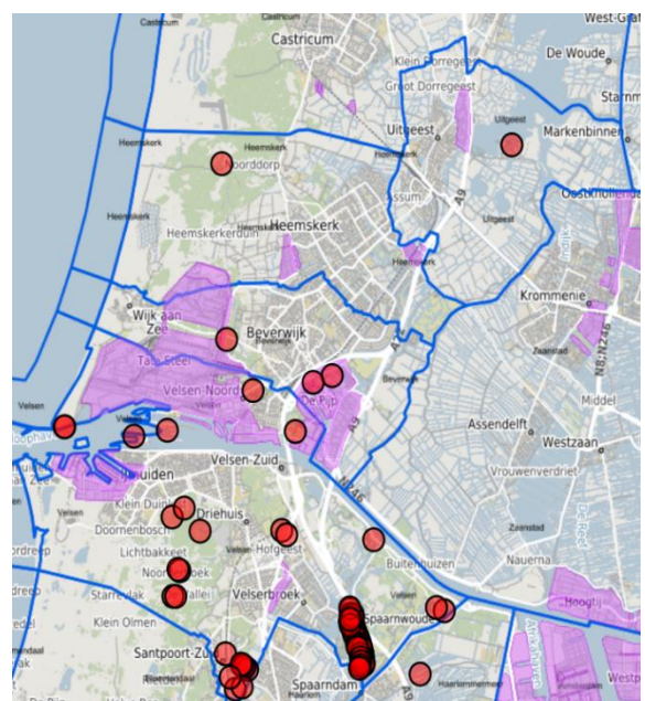
Figuur 4 – Ammoniakoelinstallatie
