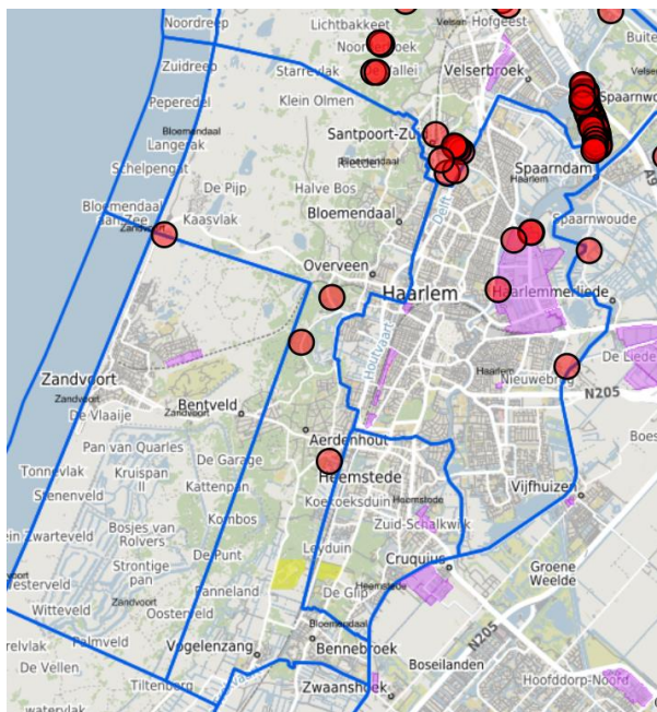
Figuur 9 – Propaantanks
